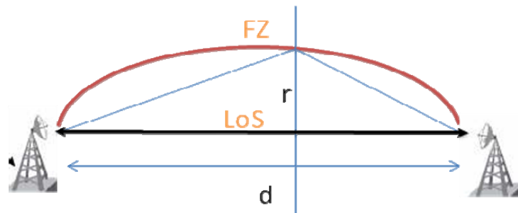
Figura 1. Cálculo de la Zona de Fresnel.
