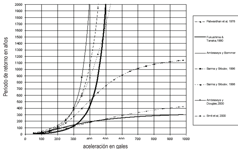
Figura 2. Curvas de Amenaza Sísmica para Tunja 1935- 2009
