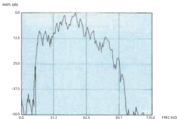
Figura 4. Trazo del geófono.
