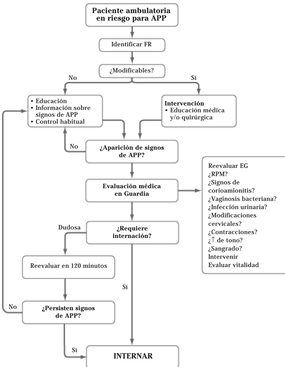
Figura 1: Algoritmo
