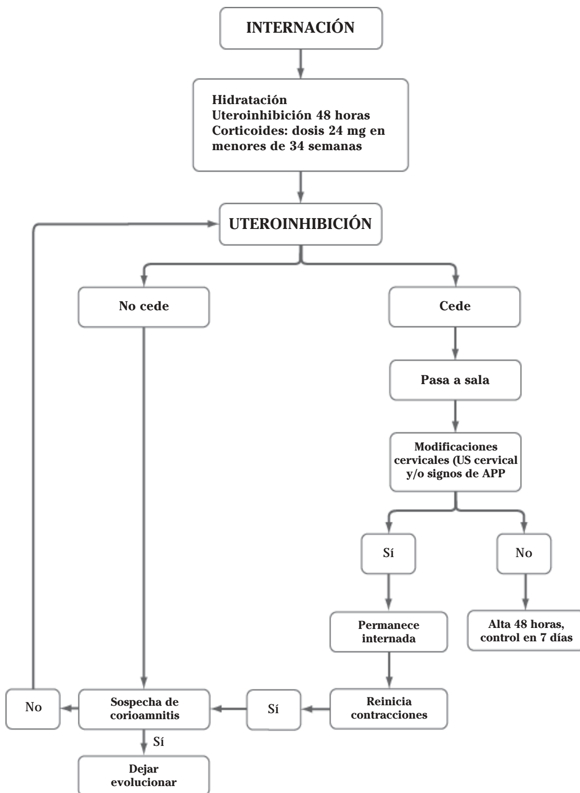
Figura 2: Algoritmo
