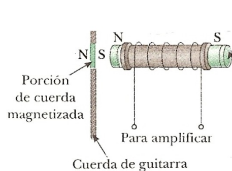
Figura 1. La cuerda vibrante induce una f.e.m. en la bobina.
