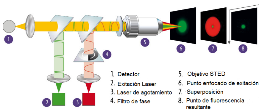
Fig. 1: Representación del funcionamiento de la tecnología STED (www.activemotif.com)
