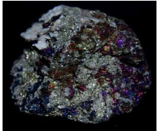
Figura 61. Calcopirita (amarilla, metálica) con pátinas muy coloreadas de bornita (lila, metálica) y covellina (azul). Butte, Montana, EUA.
