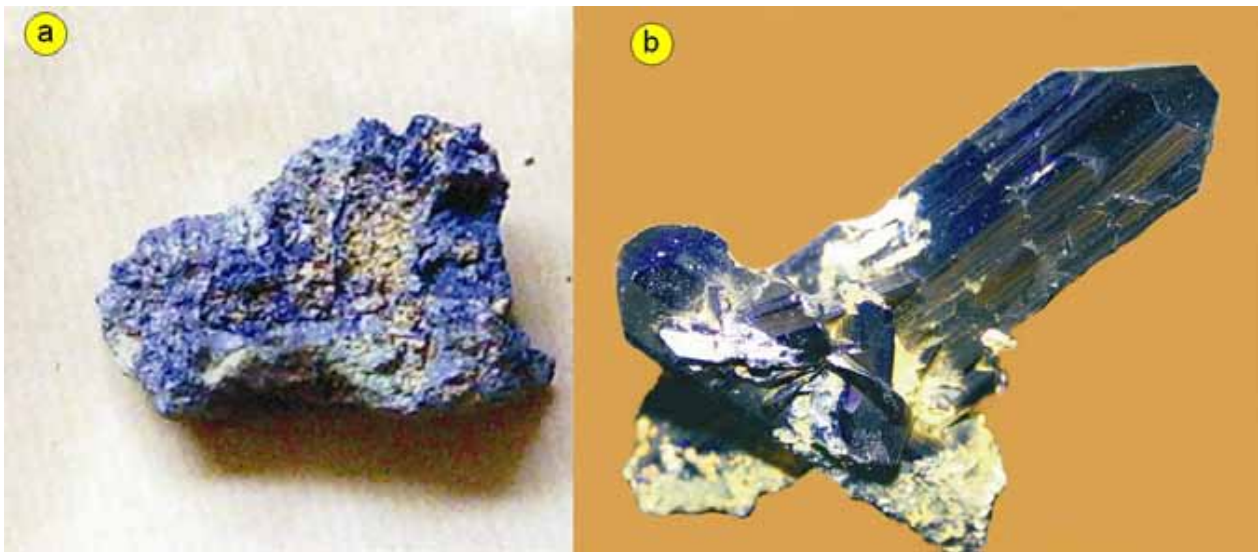
Figura 73. a) Costras de azurita microcristalina típica; b) cristales prismáticos muy bien definidos. Touisit, Marruecos
