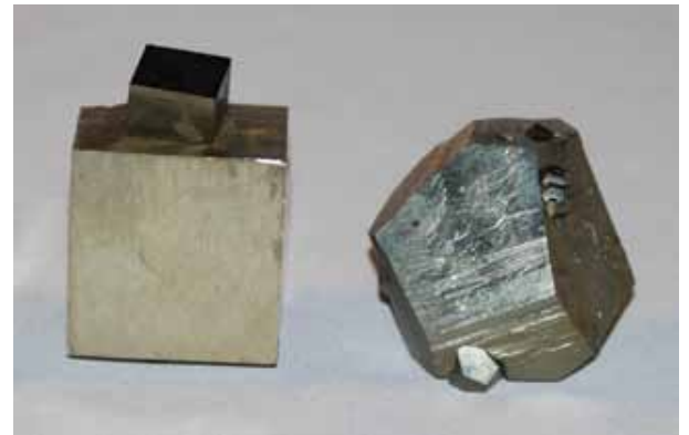
Figura 33. Formas cristalinas diferentes de la pirita: la de la izquierda es más común y la de la derecha, más rara.
