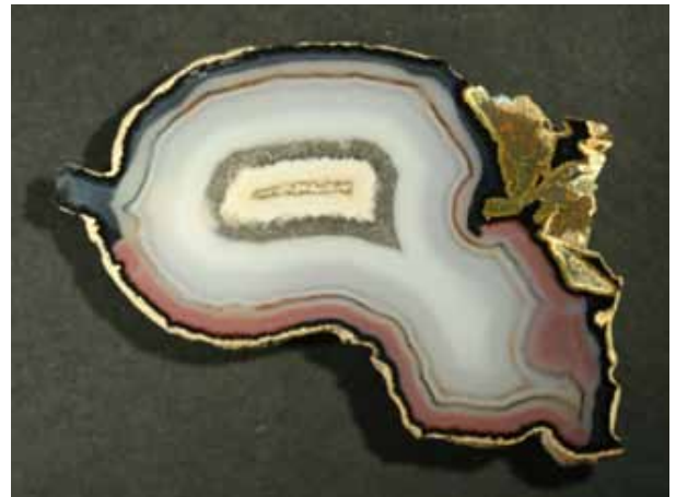
Figura 58. Crecimiento concéntrico en un ágata, en parte ya tallada y pulida.
