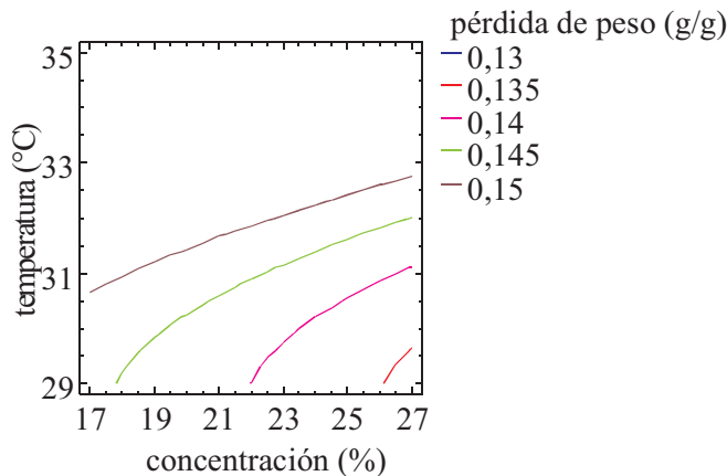
FIGURA 2. GRÁFICA DE CONTORNO DE LA PÉRDIDA DE PESO MOSTRANDO LAS CURVAS QUE MEJOR SATISFACEN EL CRITERIO DE OPTIMIZACIÓN.
