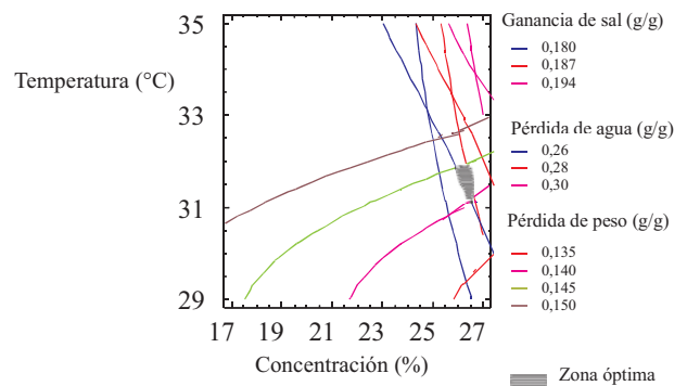
FIGURA 4. ZONA ÓPTIMA PARA LA DESHIDRATACIÓN OSMÓTICA DE LAS LÁMINAS DE SARDINA: CONCENTRACIÓN DE SALMUERA DE 26,5%; TEMPERATURA DE 31,6° A 31,8°C Y TIEMPO DE 245 min.
