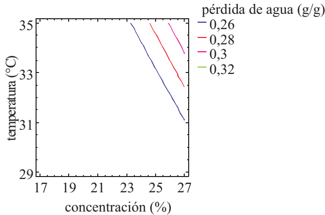
FIGURA 1. GRÁFICA DE CONTORNO DE LA PÉRDIDA DE AGUA MOSTRANDO LAS CURVAS QUE MEJOR SATISFACEN EL CRITERIO DE OPTIMIZACIÓN.
