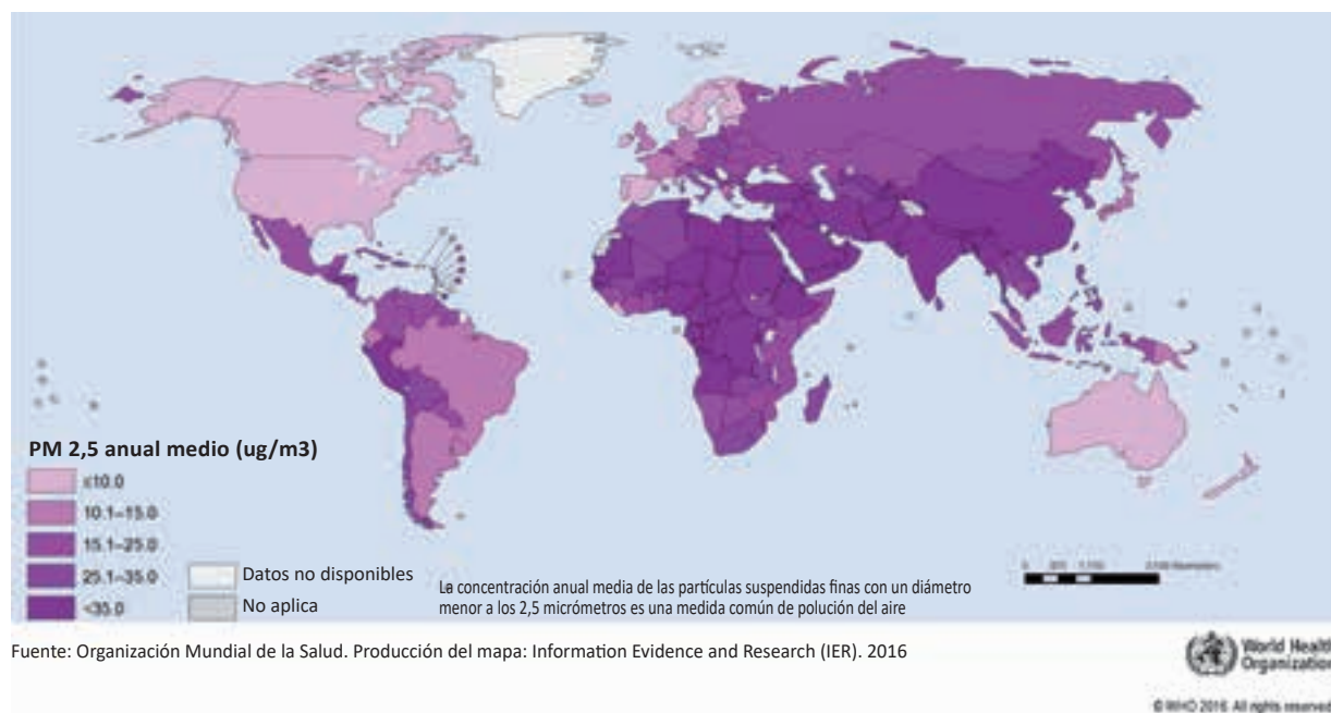
Figura 1. Concentración anual promedio de materia particulada fina (PM 2,5) en áreas urbanas ( \mu\text{g}/\text{m}^3 ), 2014.
