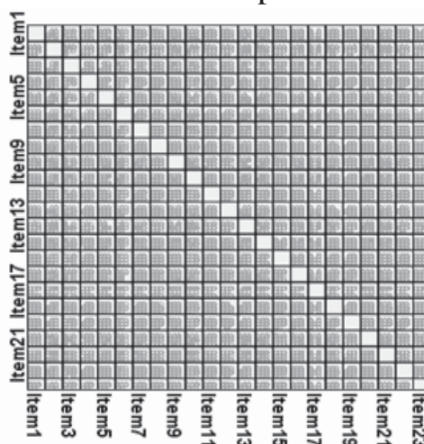
Figura 1 Gráfico de dispersión
